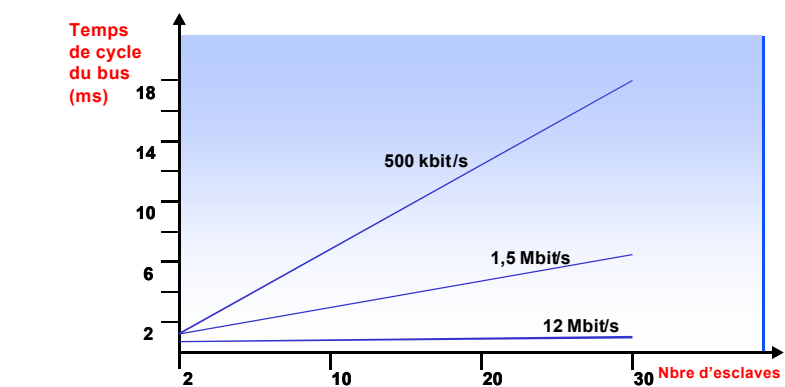
Fig. 9 : Temps de cycle du bus en configuration DP monomaître. Limite : 2 octets d'entrée et de sortie par esclave
